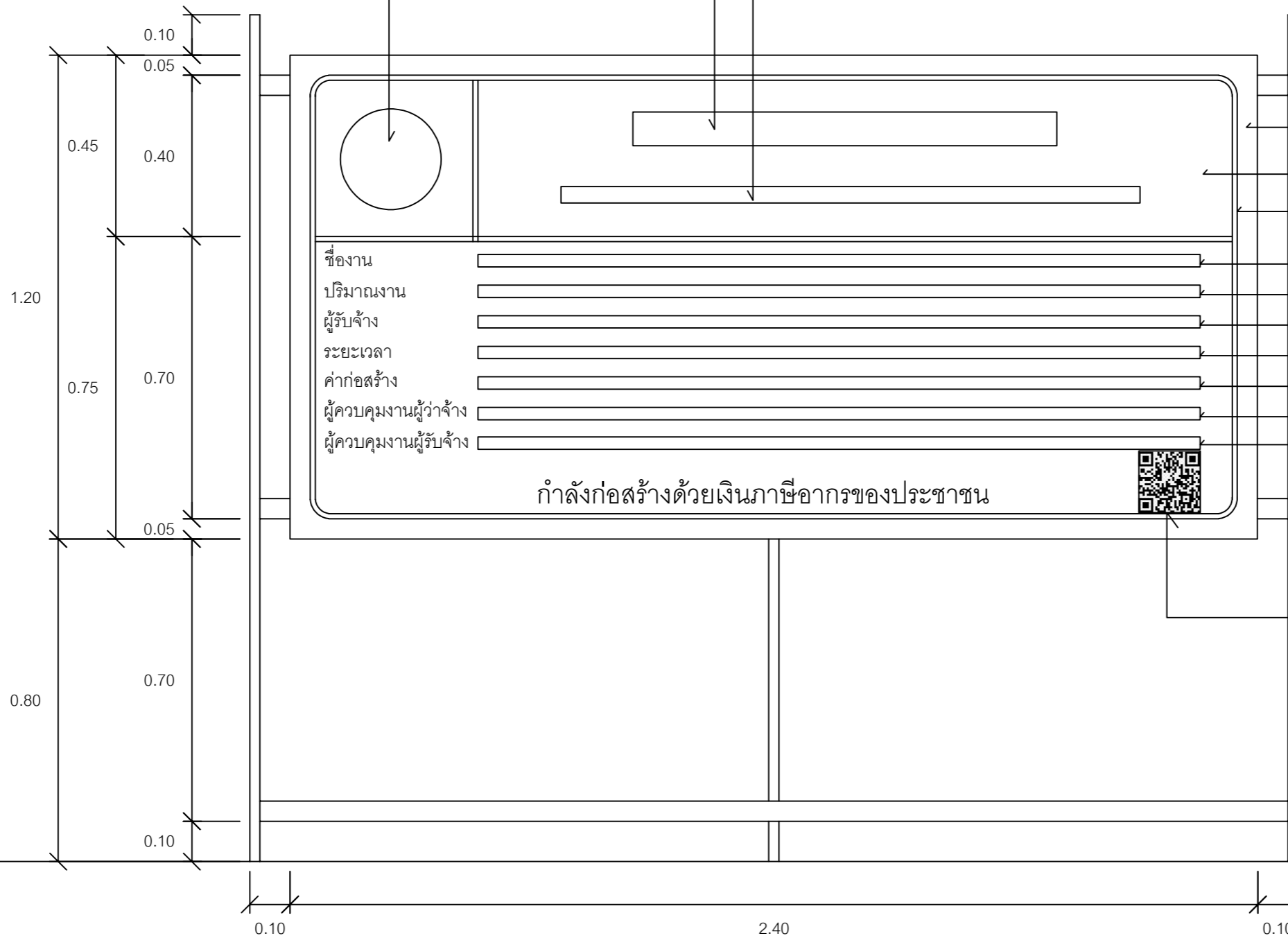
รูปด้านหน้า 1 : 50
