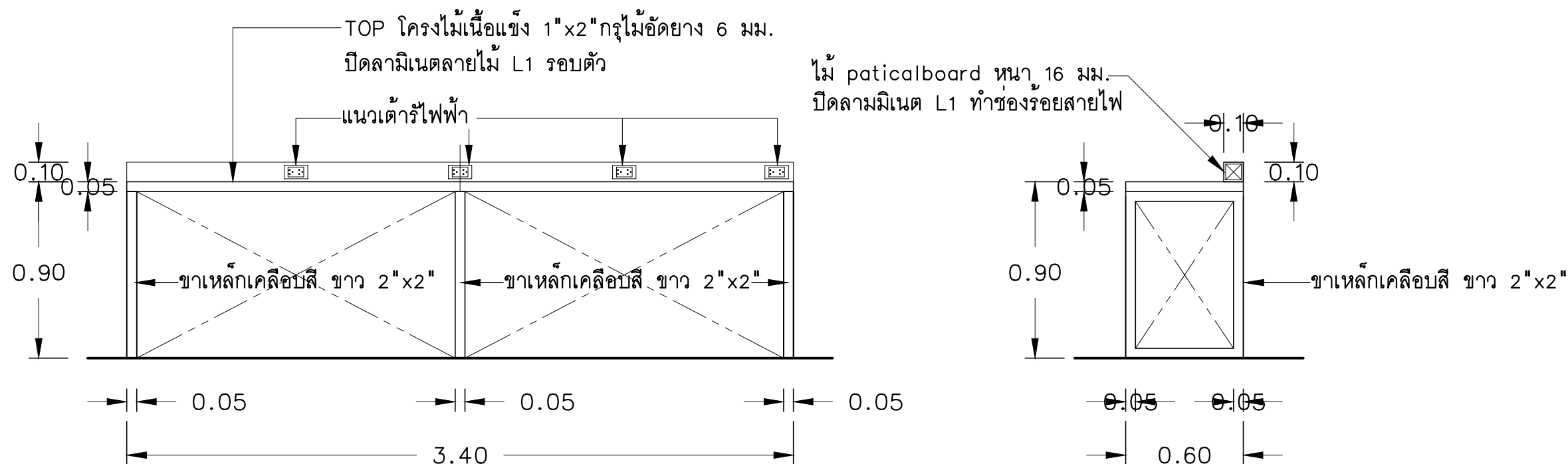
รูปด้านหน้า SCALE A1=1:25,A3=1:50
