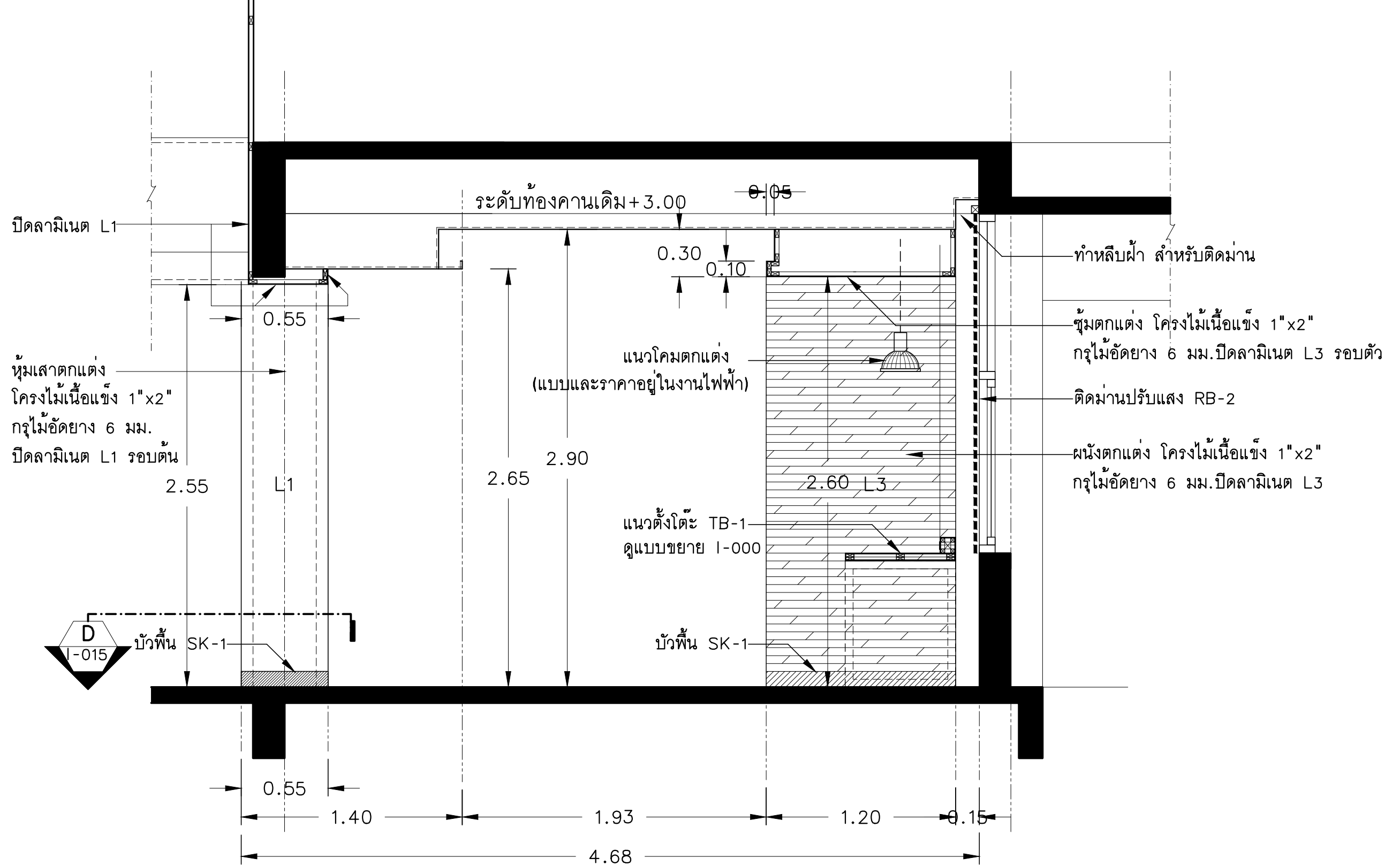
รูปตัด SCALE A1=1:25, A3=1:50
