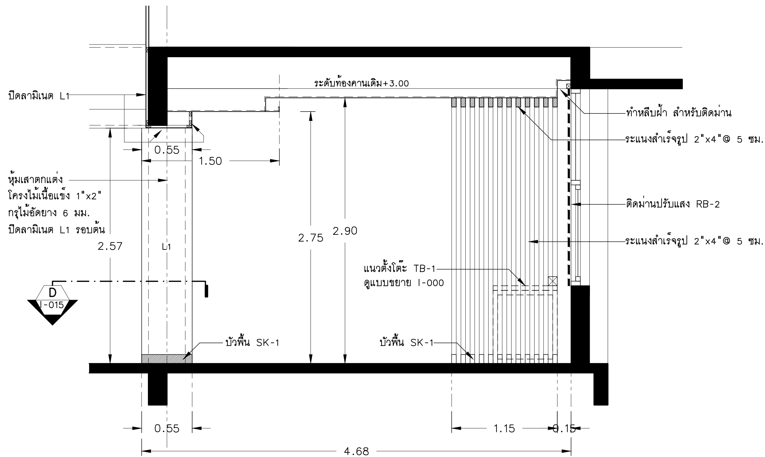
รูปตัด C SCALE A1=1:25,A3=1:50
