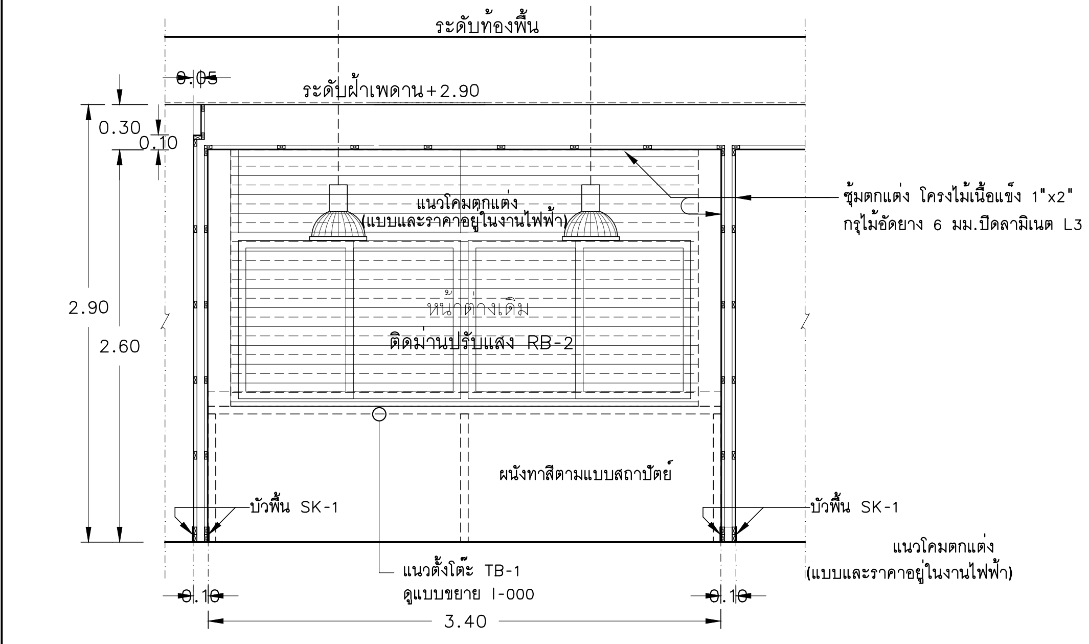
รูปตัด SCALE A1=1:25, A3=1:50
