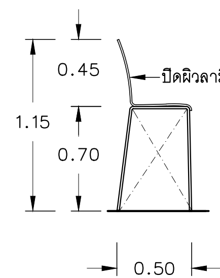
รูปด้านข้าง SCALE A1=1:25,A3=1:50
