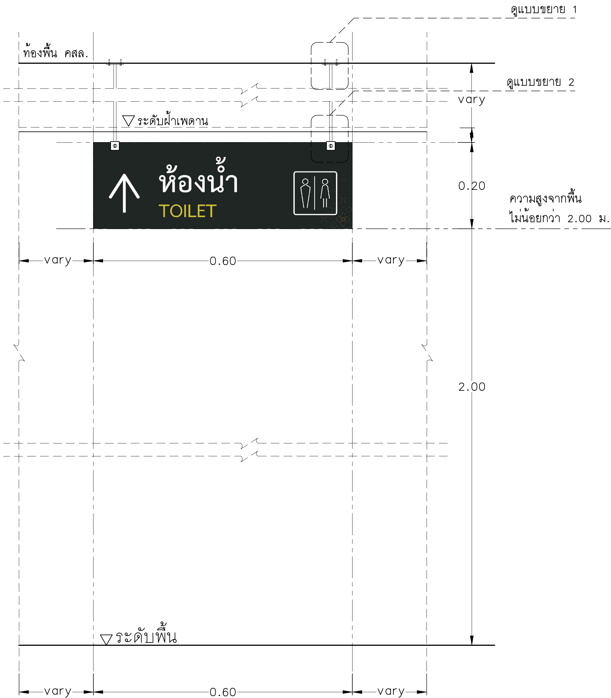
แบบขยายการติดตั้ง ป้ายแบบแขวนผ้า SCALE A3=1:10, A1=1:5
