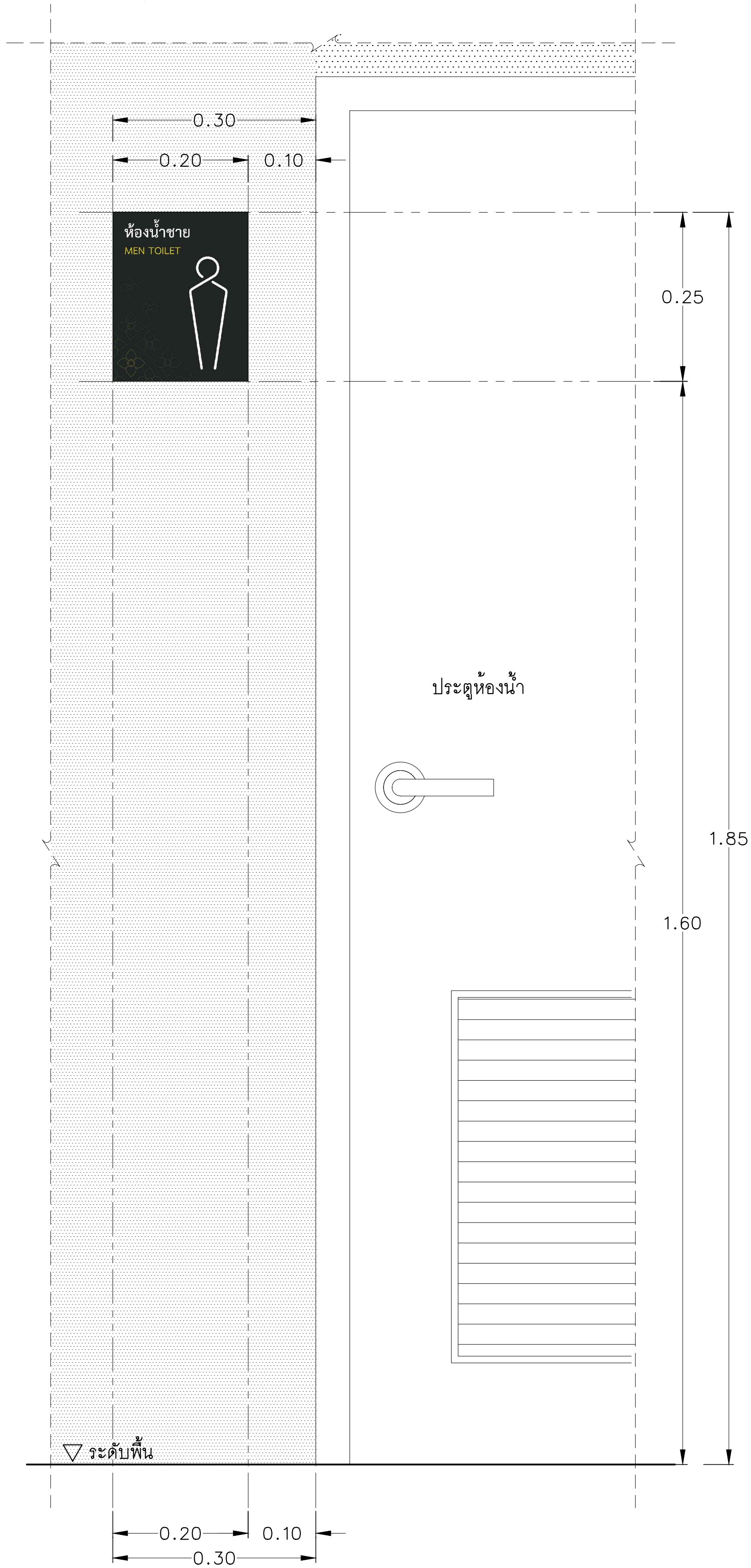
แบบขยายการติดตั้ง ป้ายห้องน้ำ SCALE A3=1:10, A1=1:5
