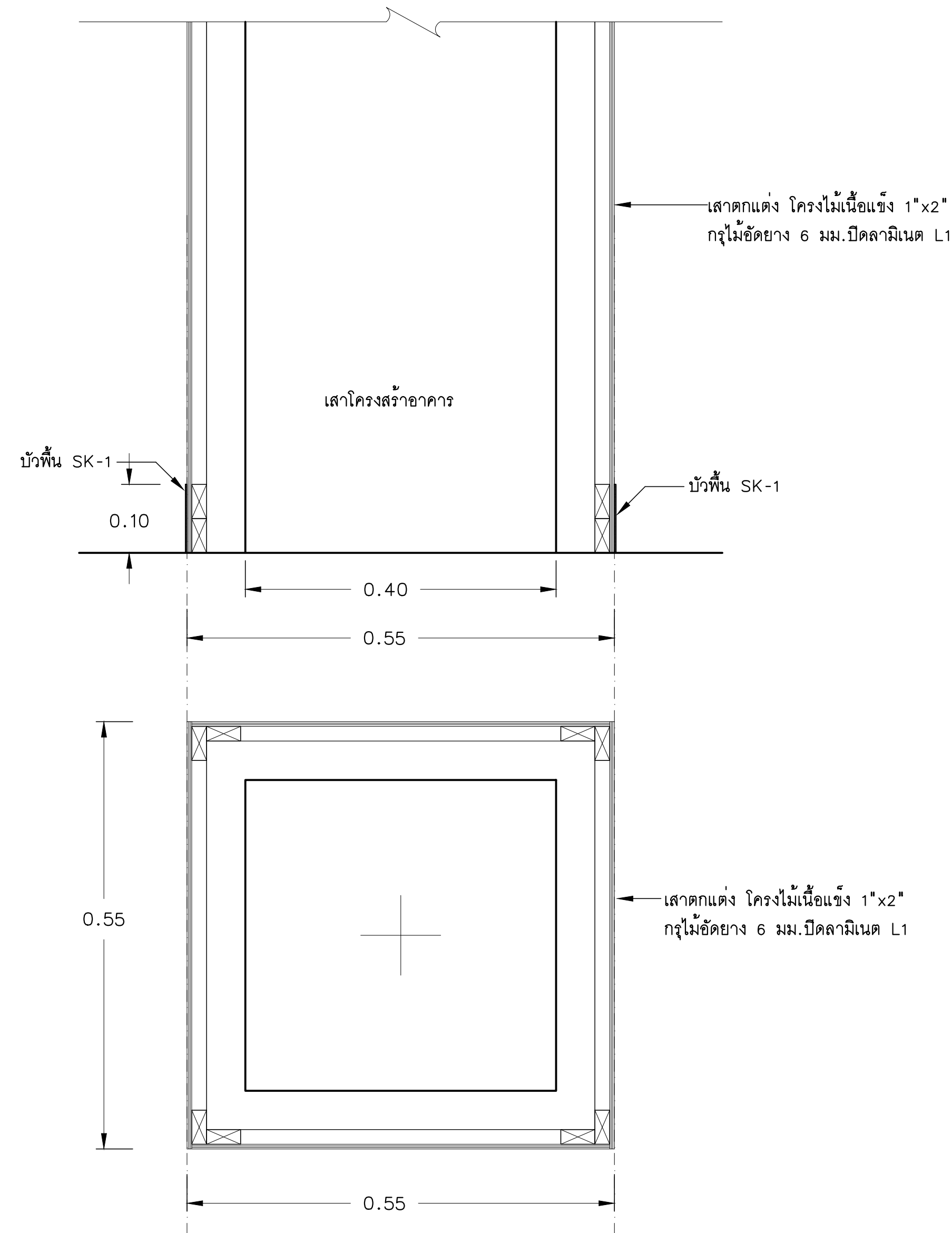
แปลน-รูปตัดขยาย SCALE A1=1:5,A3=1:10
