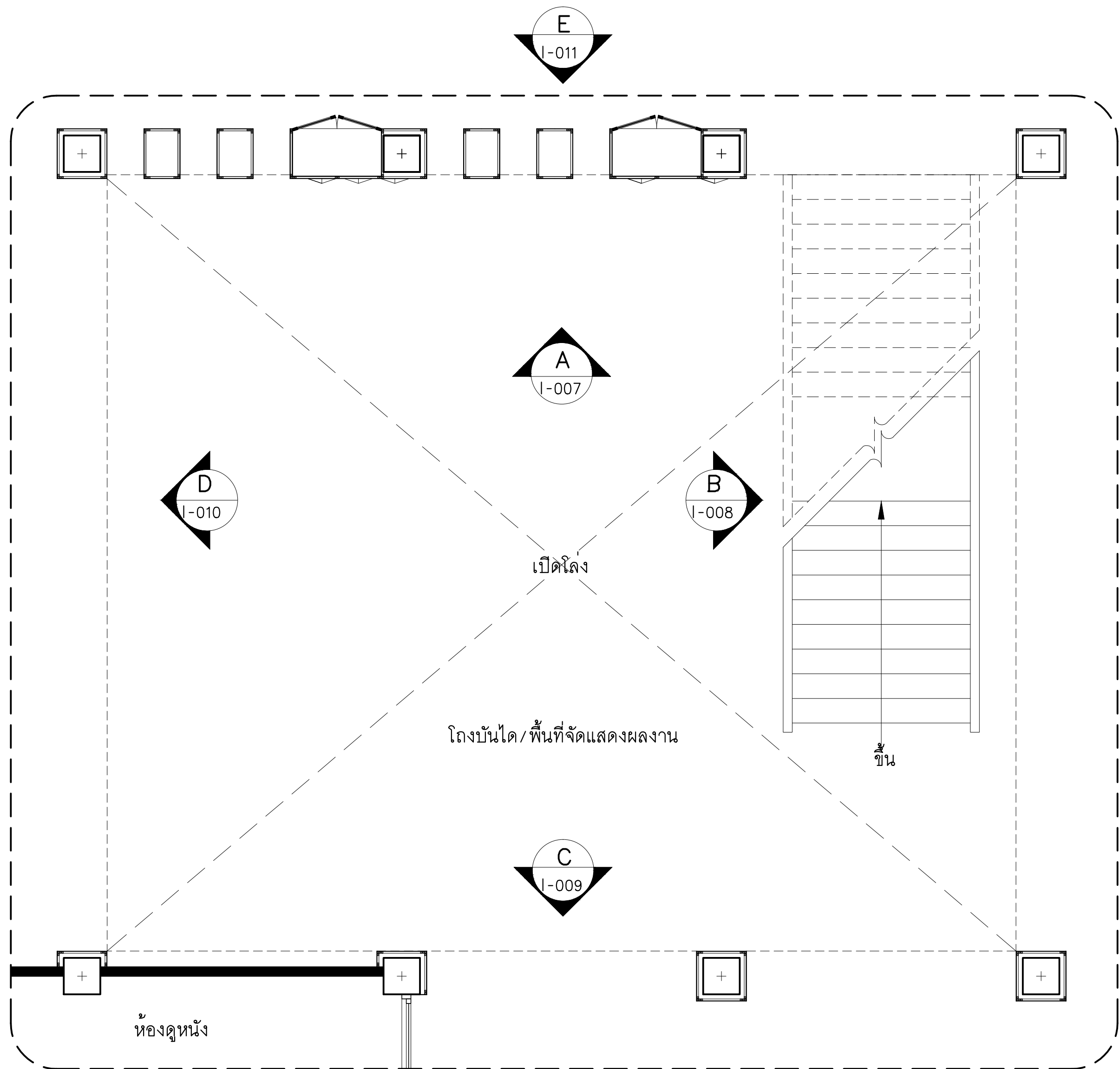
แปลนขยายโถงบันได/พื้นที่แสดงนิทรรศการ ชั้น 1 มาตราส่วน A3=1:75,A1=1:37.5
