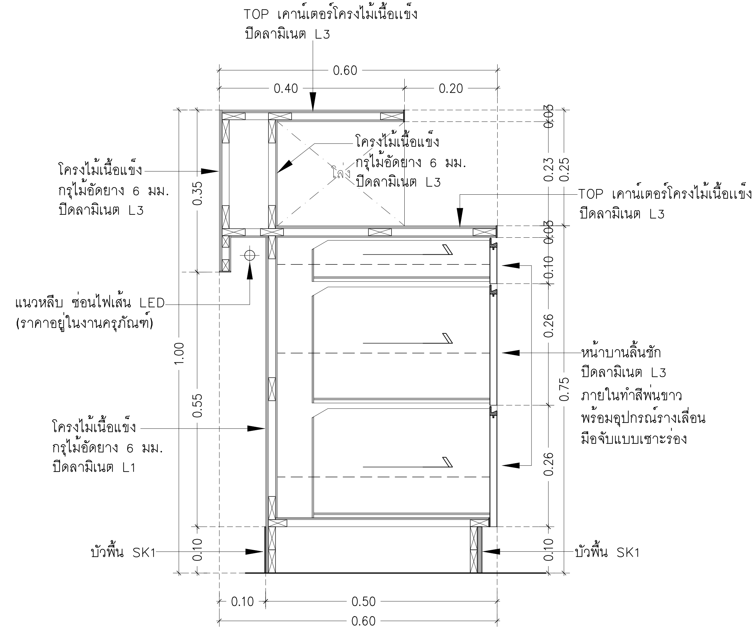
2 รูปตัด I-017 มาตรฐาน A3=1:10, A1=1:5
