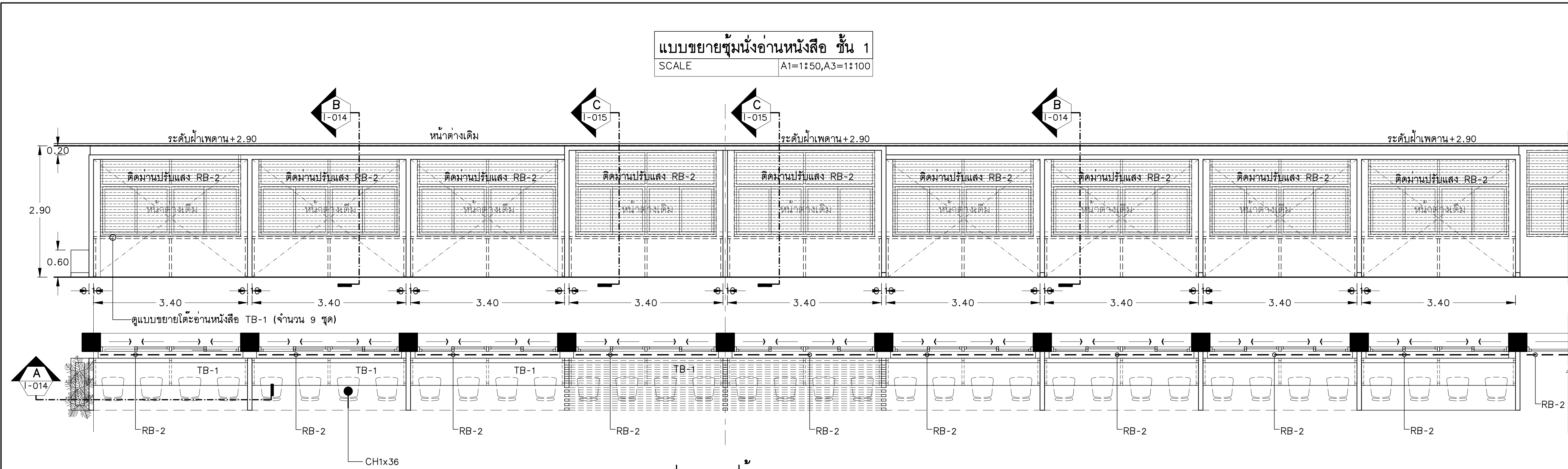
แปลน - รูปด้าน มาตราส่วน A1=1:50, A3=1:100
