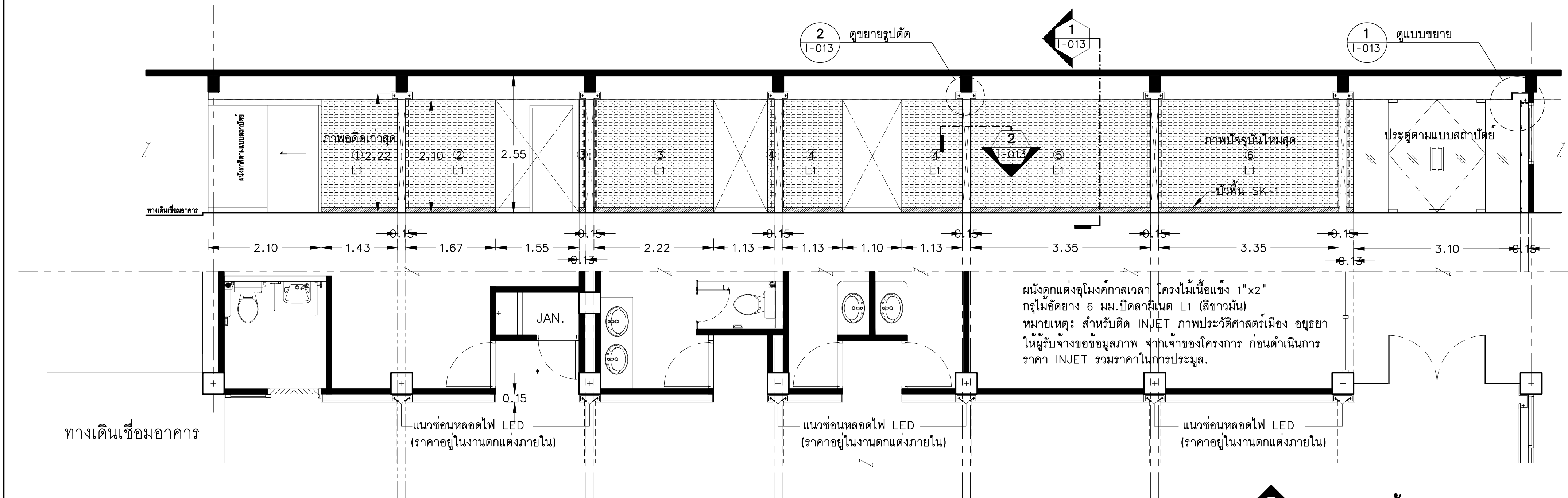
A แปลน-รูปด้าน I-012 / มาตราส่วน A3=1:100, A1=1:50
