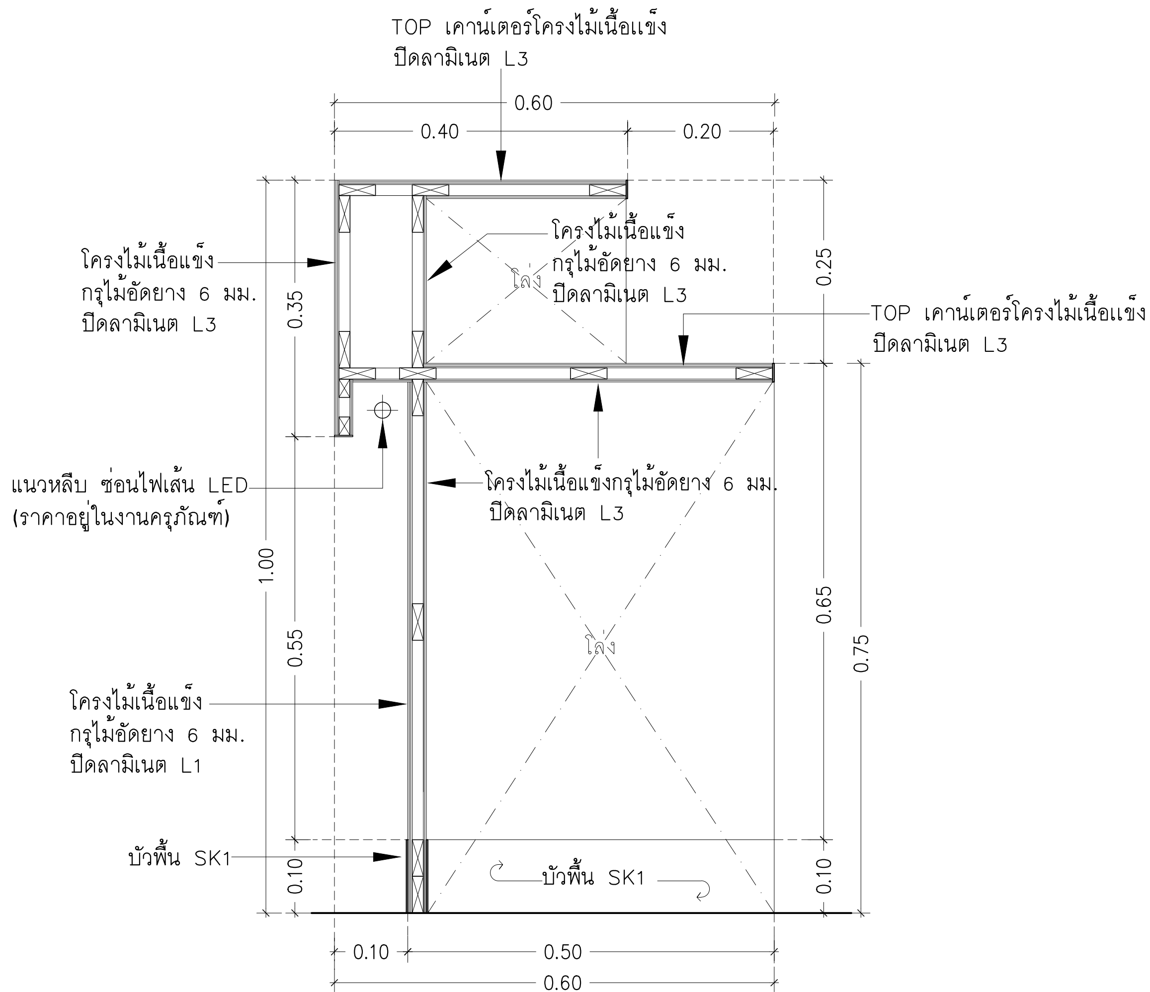
2 รูปตัด I-017 มาตรฐาน A3=1:10, A1=1:5
