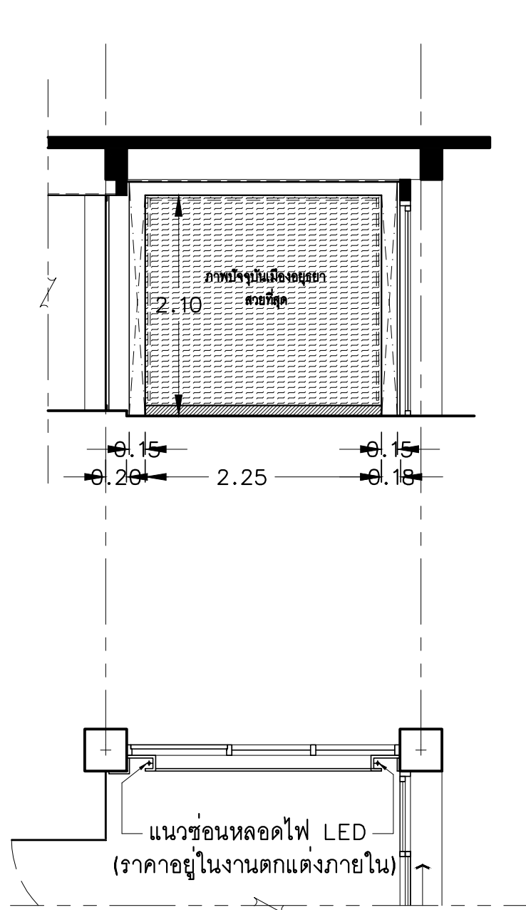
C แปลน-รูปด้าน I-012 / มาตราส่วน A3=1:100, A1=1:50
