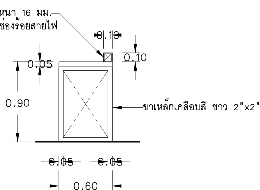
รูปด้านข้าง SCALE A1=1:25,A3=1:50
